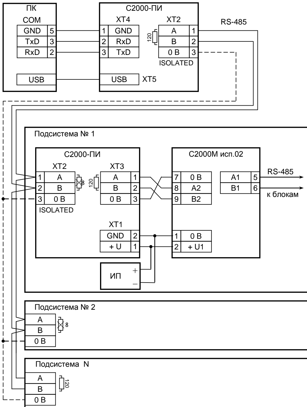
С2000М исп.02 – пульт контроля и управления «С2000М исп.02»; С2000-ПИ – преобразователь-повторитель интерфейсов «С2000-ПИ»; ИП – резервированный источник питания.
