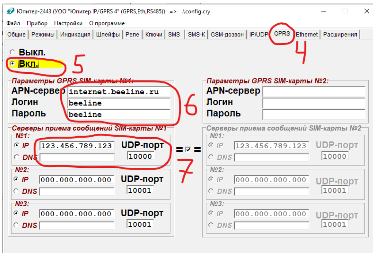
Рисунок 6.38 Настройка прибора для работы по GPRS
