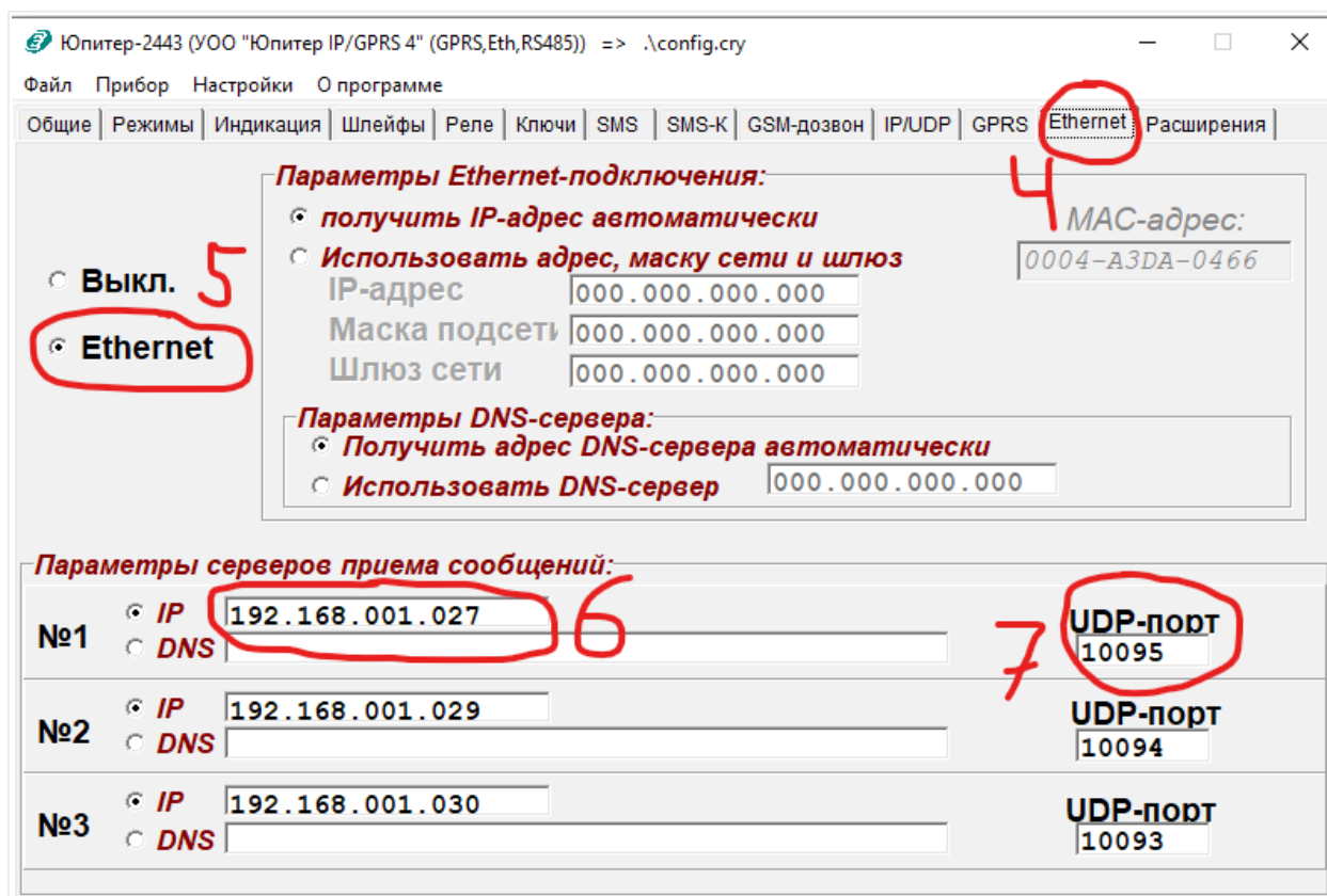
Рисунок 6.37 Настройка прибора для соединения по Ethernet
