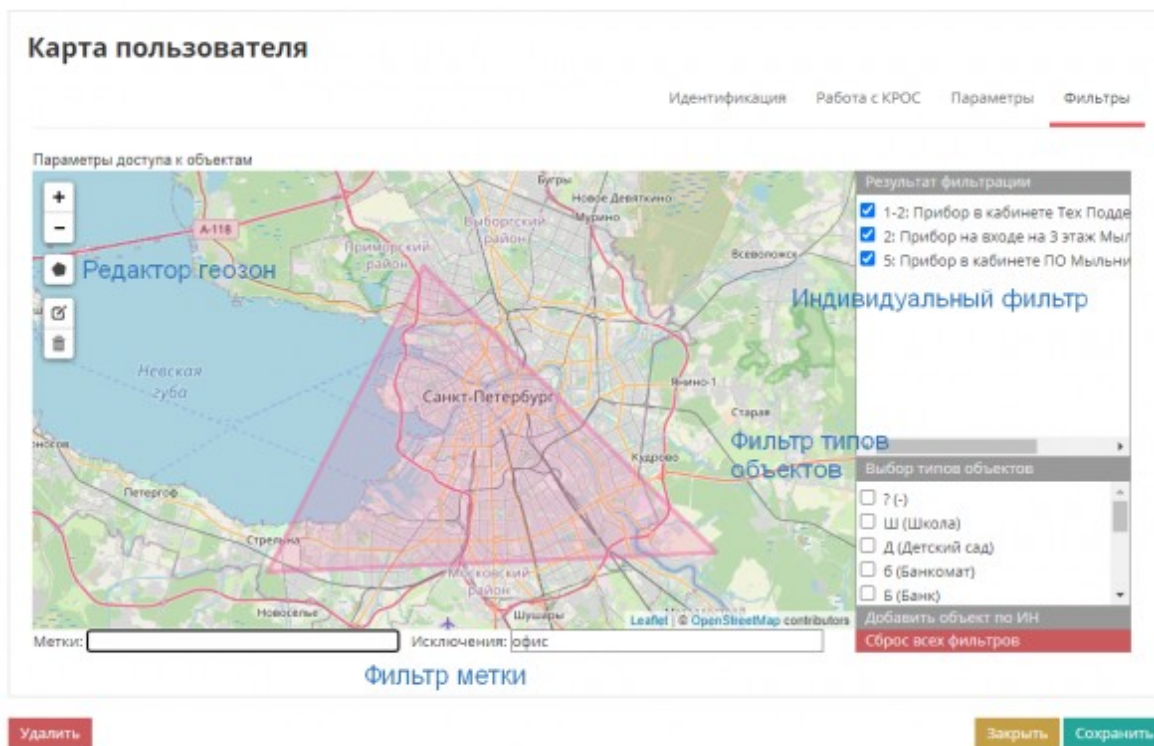
Рисунок 7.10 Окно фильтра объектов
