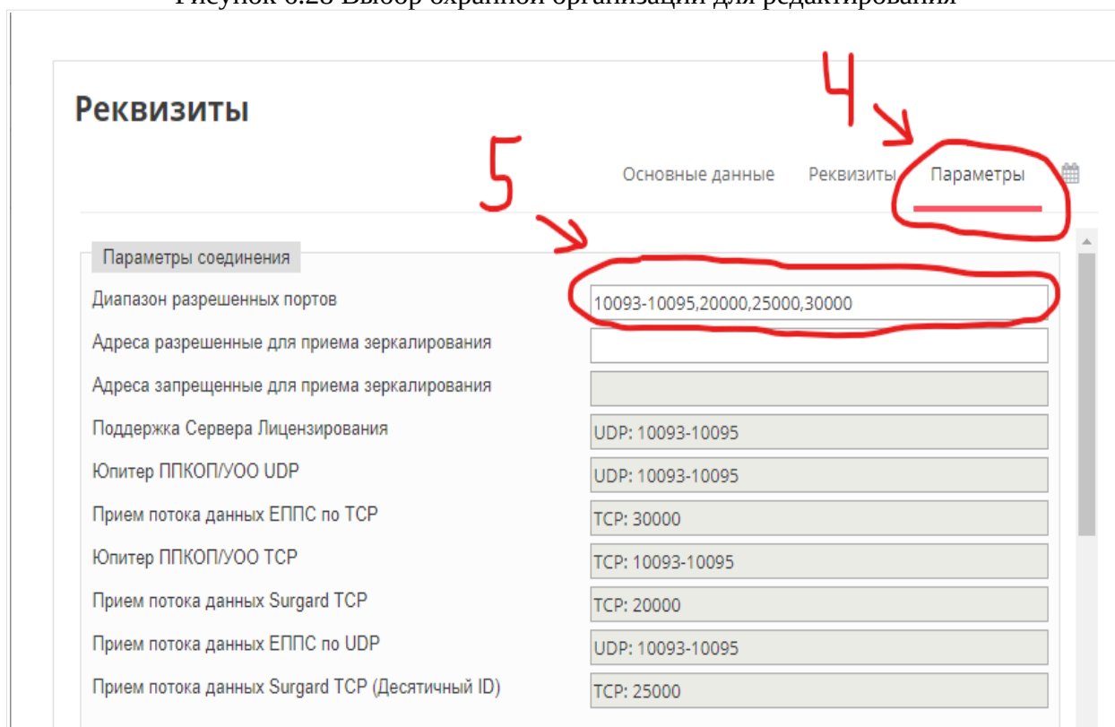
Рисунок 6.29 Редактирование данных для охранной организации
