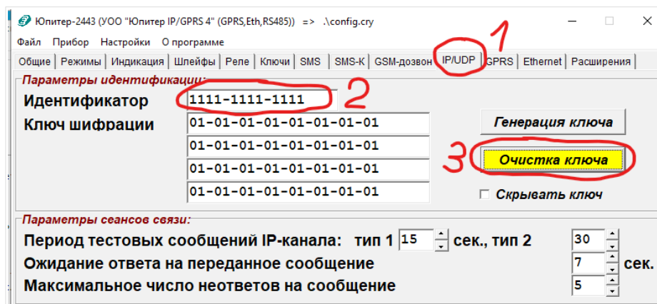
Рисунок 6.36 Настройка IP/UDP
