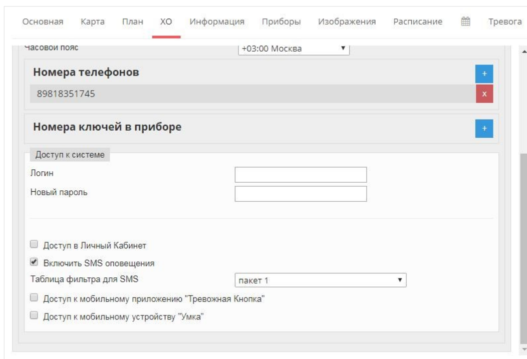
Рисунок 7.5 Включение СМС-оповещений для SMPP сервера
