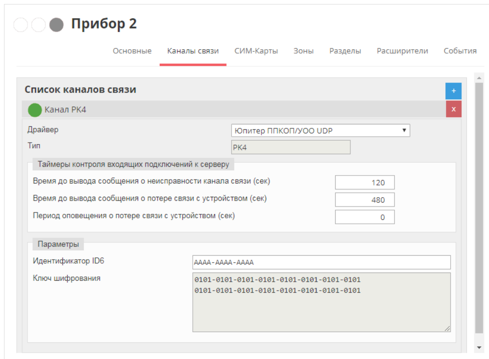
Рисунок 6.19 Вкладка «Каналы связи»
