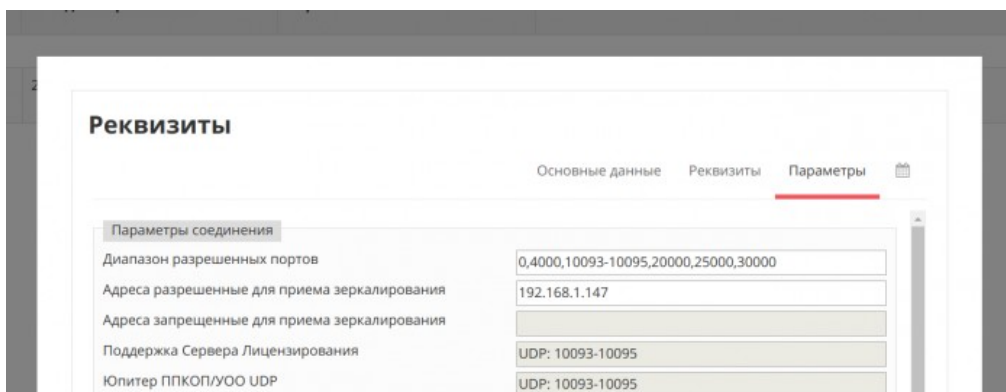
Рисунок 9.2 Разрешение приема данных
