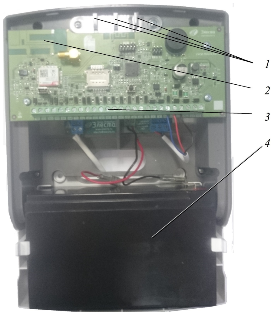
Рисунок 2.1. Прибор Сатурн-2819 с открытой крышкой
