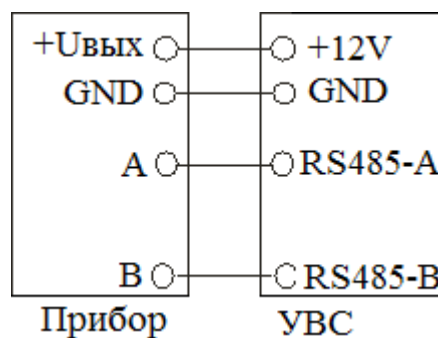
Рисунок 3.5. Подключение УВС по RS485
