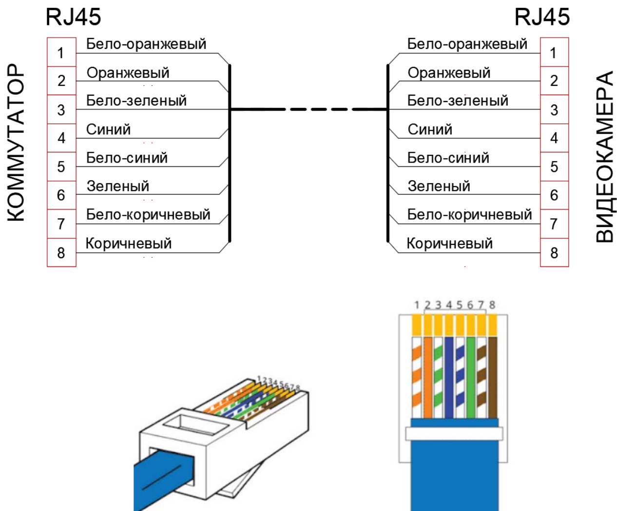
Рисунок 13. Разделка кабеля витая пара
