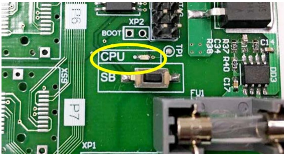
Рисунок 10. Расположение элементов индикации и настройки на плате коммутатора
