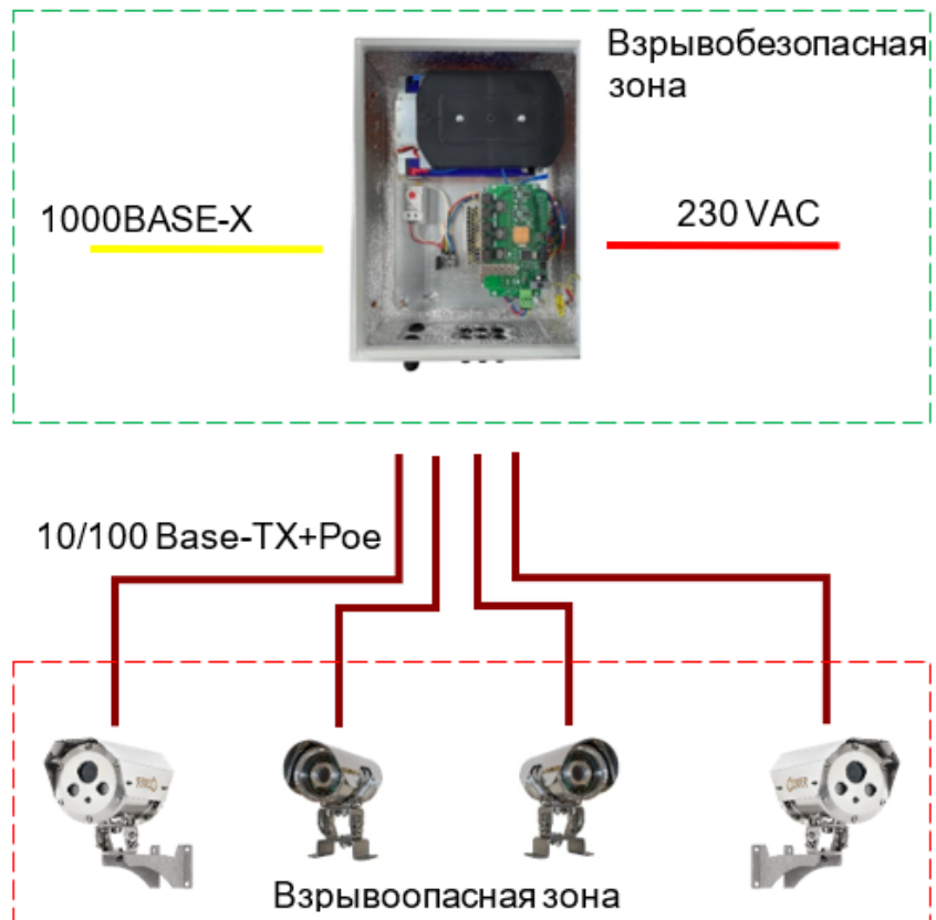
Рисунок 2. Типовая схема подключения коммутатора по оптическому кабелю для работы с взрывозащищенным оборудованием
