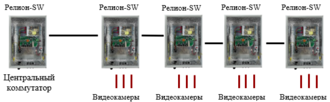
Рисунок 8. Подключение коммутаторов в топологию «линия»
