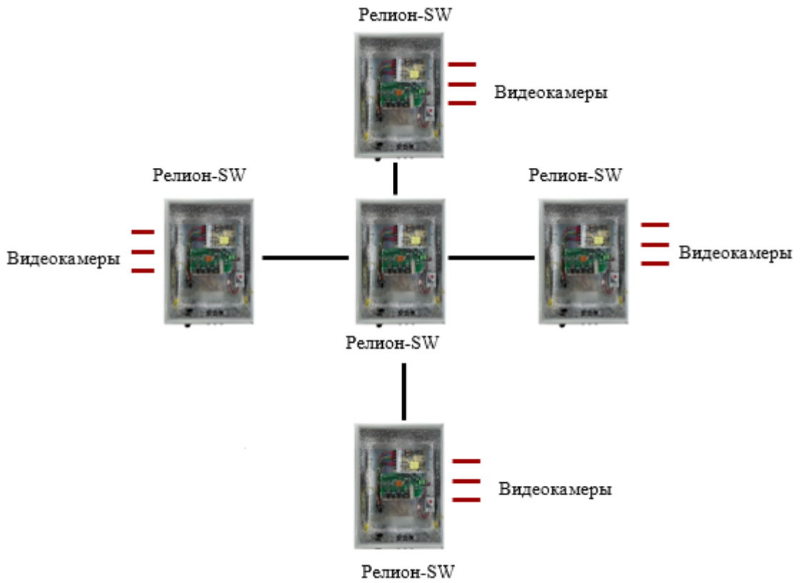
Рисунок 7. Подключение коммутаторов в топологию «звезда»
