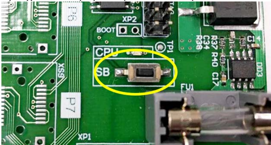
Рисунок 11. Кнопка для принудительной перезагрузки коммутатора
