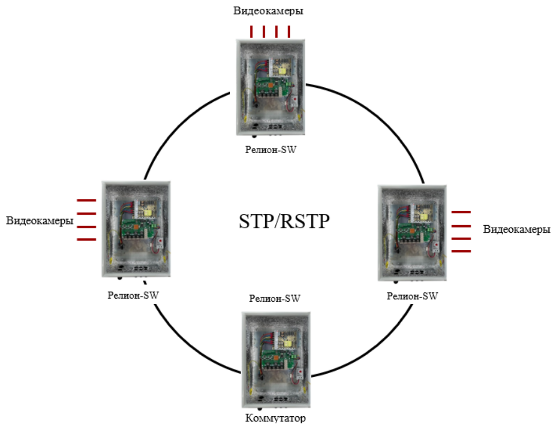
Рисунок 9. Подключение коммутаторов в топологию «кольцо»
