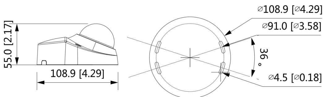
Рисунок 5.1 – Габаритные размеры видеокамеры
