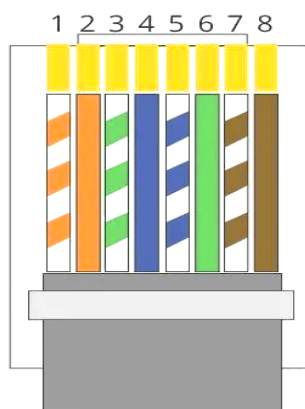
Рисунок 5.3 – Штекер 8P8C
