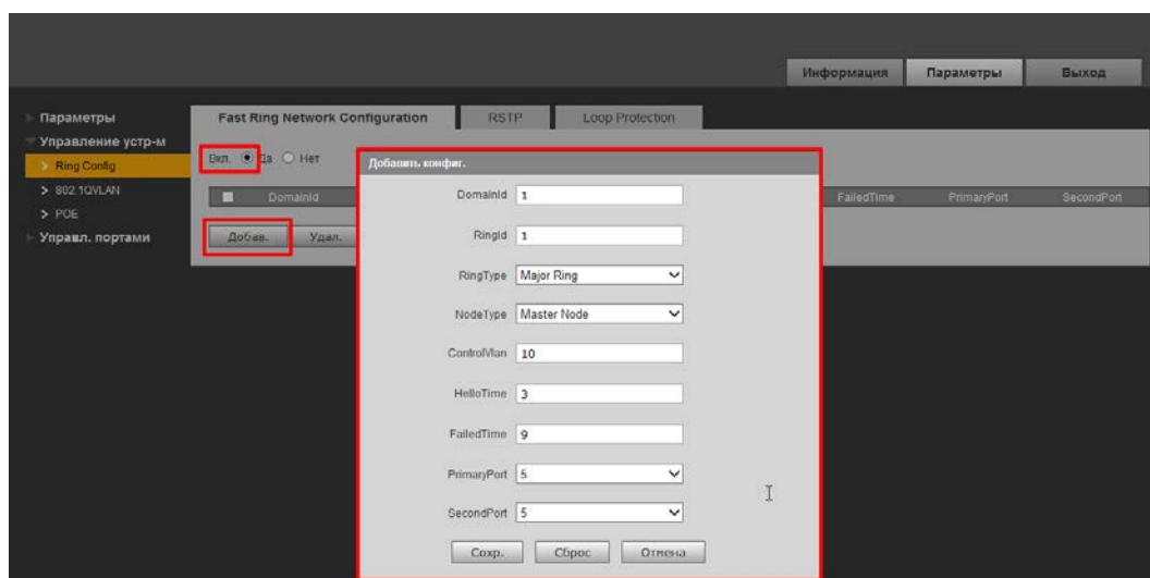
Рисунок 6.9 – Настройка конфигурации сети
