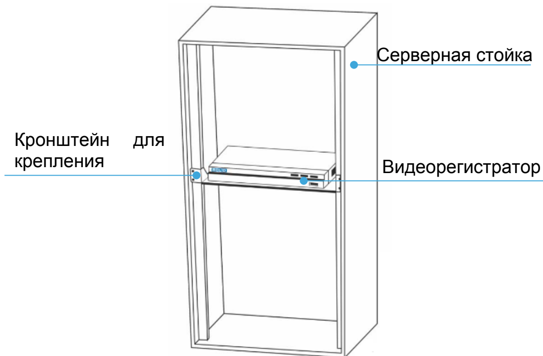
Рисунок 3.11 – Монтаж видеорегистратора в 19” - стойку с помощью кронштейна
